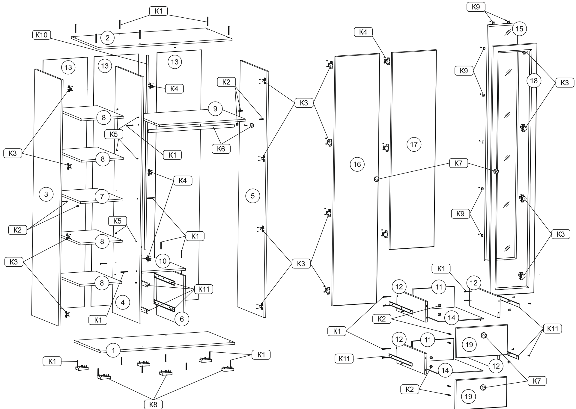
Схема 1. Сборка шкафа
