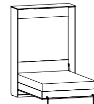
Арт. K01 Шкаф-кровать 1541x495, h 2216 мм (в сложенном виде) 1541x2250, h 2216 мм (в разложенном виде) Спальное место: 2000x1400 мм (можно дополнить зеркалом Арт. ЗК01)
