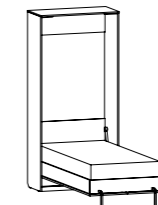
Арт. K02 Шкаф-кровать 1041x490, h 2216 мм (в сложенном виде) 1041x2250, h 2216 мм (в разложенном виде) Спальное место: 2000x900 мм (можно дополнить зеркалом Арт. ЗК01)
