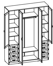
Арт. 112 Шкаф для белья со штангой, полками и ящиками 1640×490, h 2216 мм (можно дополнить зеркалом Арт. 3100)
