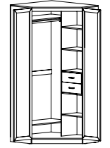
Арт. 403 Шкаф угловой со штангой, полками и двумя ящиками 942+1062(угол)×490(слева)/370(справа), h 2216 мм (универсальная схема сборки, можно дополнить зеркалом Арт. 3100)
