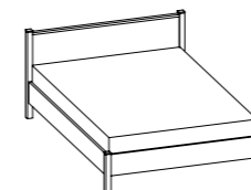
Арт. 612/614/615/616 Кровать с ортопедическим основанием 2090x990/1490/1690/1890, h 922 мм Спальное место: 2000x900/1400/1600/1800 мм
