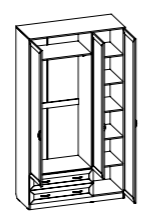
Арт. 114 Шкаф для белья со штангой полками и ящиками 1230×490, h 2216 мм
