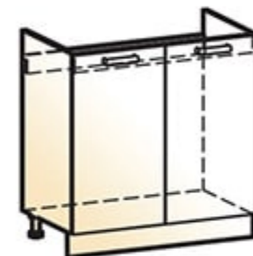
42 Шкаф рабочий под мойку (2 двери) → | 7 | ↑ 800|456|820
