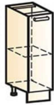
47 Шкаф рабочий (1 дверь) → | 7 | ↑ 200|460|820
