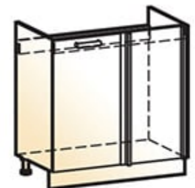
43 Шкаф рабочий под мойку угловой (1 дверь) → | 7 | ↑ 800|486|820
