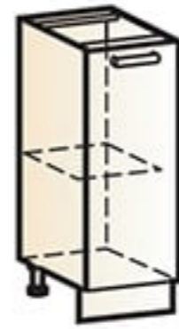
31 Шкаф рабочий (1 дверь) → | 7 | ↑ 300|460|820
