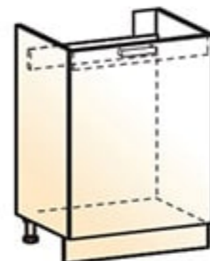
57 Шкаф рабочий под мойку (1 дверь) → | 7 | ↑ 600|456|820
