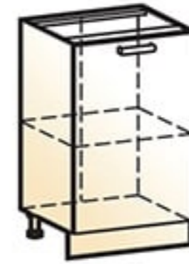
46 Шкаф рабочий (1 дверь) → | 7 | ↑ 500|460|820
