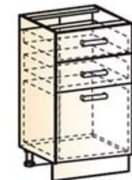
37 Шкаф рабочий (3 ящика) → | 7 | ↑ 400|460|820
