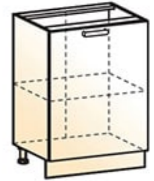
53 Шкаф рабочий (1 дверь) → | 7 | ↑ 600|460|820
